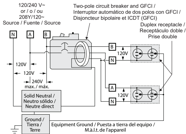
FIG. 2 : Three-wire 120/240 V or 208 Y/120V Circuits / Circuitos de 3 hilos de 120/240 V~ o 208Y/120 V~ / Circuits à 3 fils de 120/240 V ou 208Y/120 V
